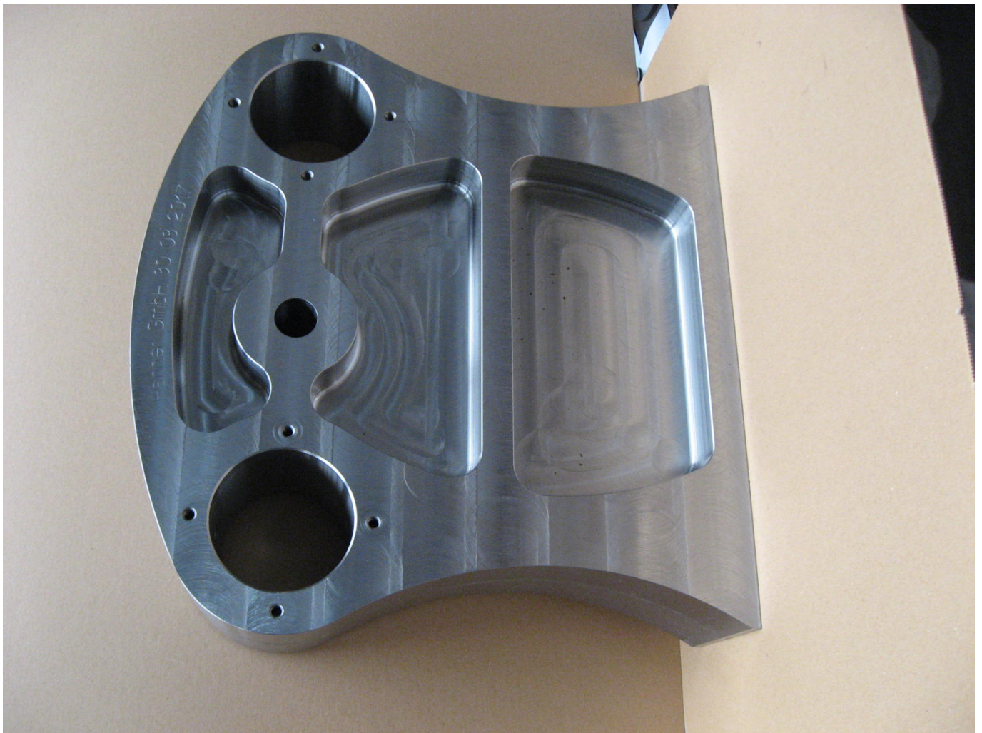
Stehlager aus St360 Dicke 116mm
