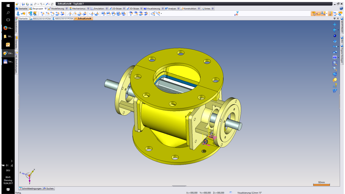
Zellradschleuse geteilt mit Verschleißeinatz
